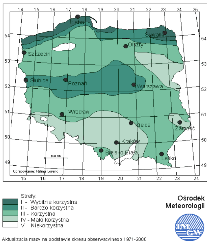
Rycina 13. Strefy energetyczne wiatru w Polsce
