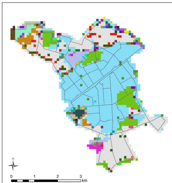
Rysunek 31. Mapa jednostek topoklimatycznych Wołomina
