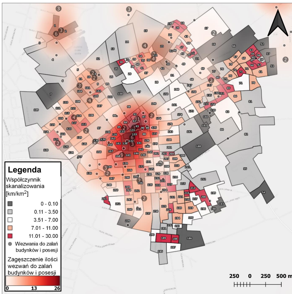
Rysunek 25. Porównanie HEAT MAP wezwań interwencyjnych straży pożarnej do podtopień z mapą współczynnika rozwinięcia sieci kanalizacyjnej
