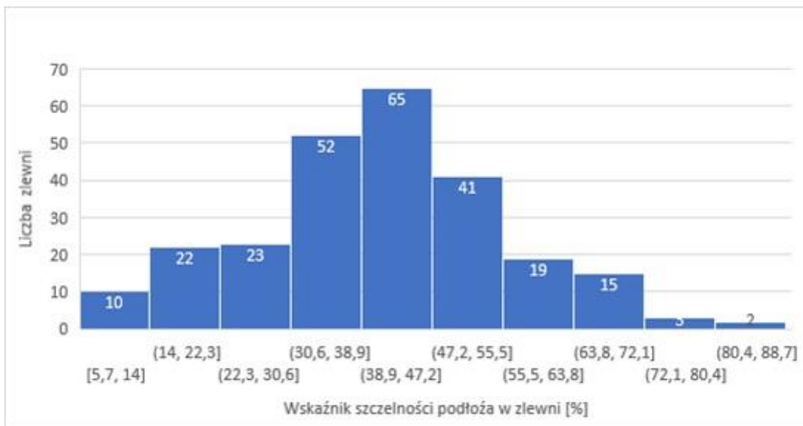
Rysunek 15. Wskaźnik szczelności podłoża w zlewniach elementarnych kanalizacji deszczowej miasta Wołomin ujętego w modelu odpływu kanalizacji burzowej
